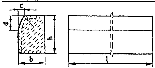
Rys. 1. Wymiarowanie krawężników
