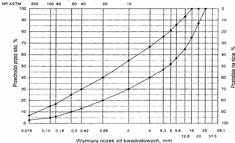
Rys. 3. Krzywe graniczne uziarnienia mieszanki mineralnej BA od 0 do 20 mm do warstwy wiążącej, wyrównawczej i wzmacniającej nawierzchni drogi o obciążeniu ruchem KR1 lub KR2
